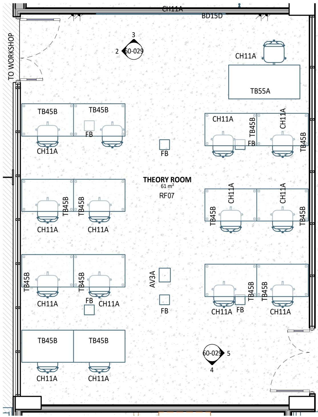
1 PLAN DETAIL 1 : 50
